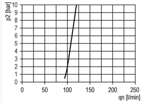
Öleransprechgrenze
